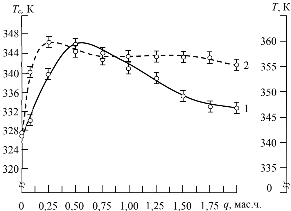
Рисунок 3 – Залежність теплофізичних властивостей епоксидної матриці від вмісту модифікатора ДААБКК: 1 – температура склування ( T_c ); 2 – теплостійкість ( T )
