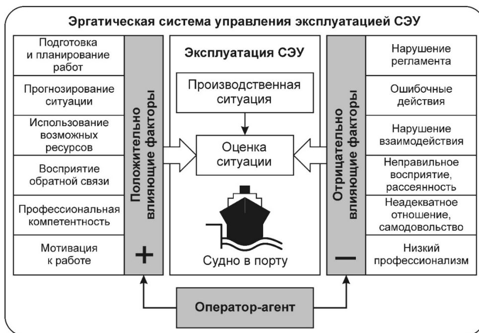
Рисунок 5 – Факторы, влияющие на объективную оценку агентом ситуации, связанной с эксплуатацией СЭУ, при стоянке судна в порту
